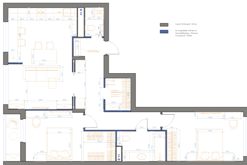
Трехкомнатная квартира. 83,5м2
